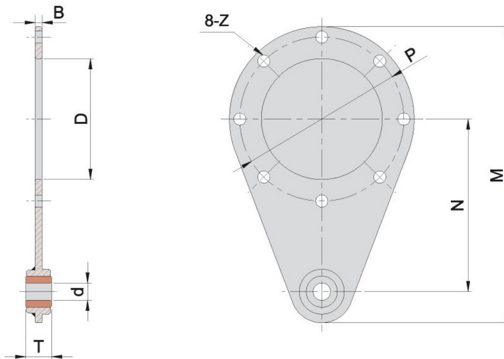
扭力臂 Torque Arm
