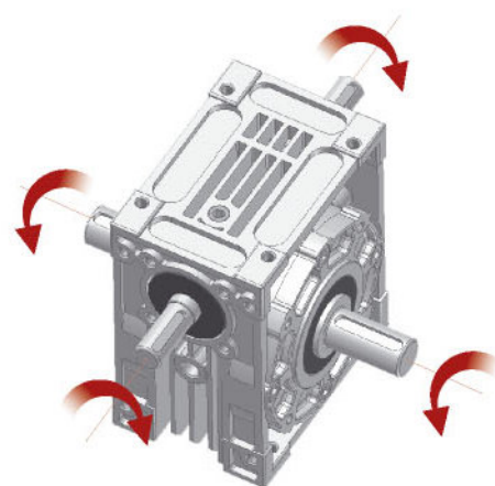
旋轉方向 Rotation Direction
